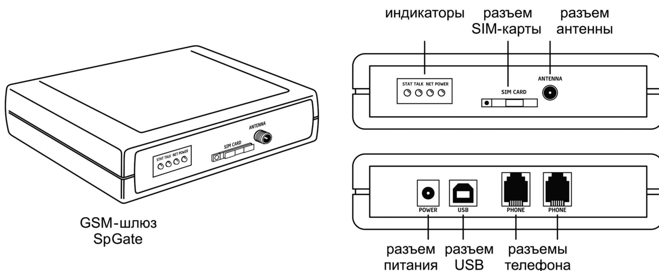
Рисунок 2.1. GSM-шлюз SpGate
