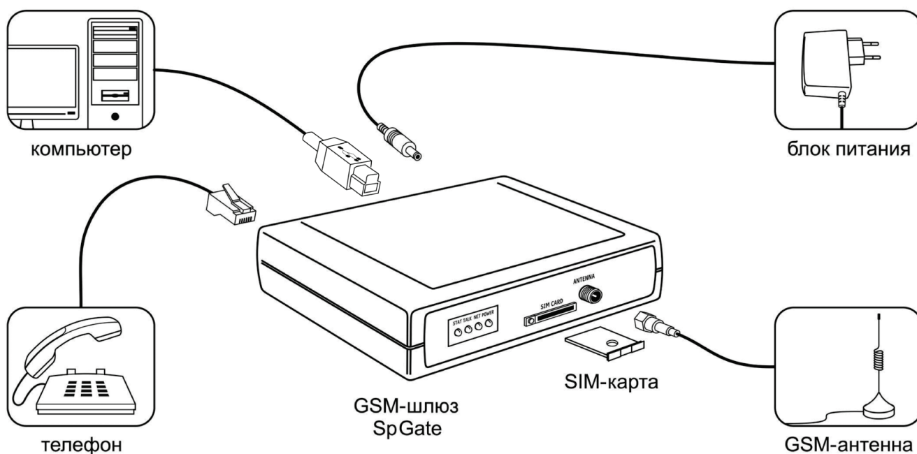
Рисунок 6.1. Подключение шлюза SpGate
