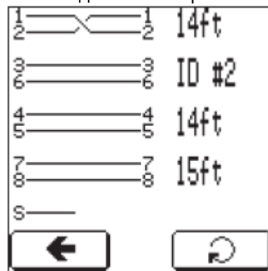
Разводка проводов с обратным подключением пары 1-2 и отсоединенным экраном.
