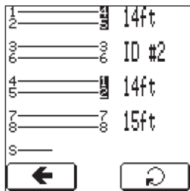
Разводка проводов с перекрещиванием проводов пар 1-2 и 4-5 и отсоединенным экраном.
