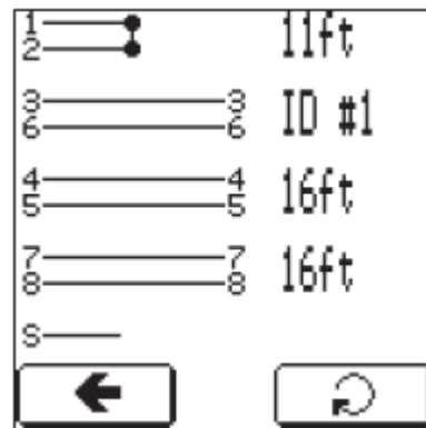
Разводка проводов с коротким замыканием на расстоянии 11 футов на паре 1-2 и отсоединенным экраном.
