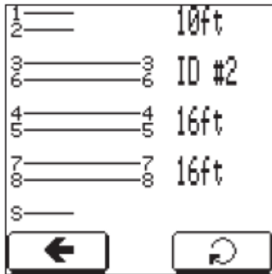
Разводка проводов с обрывом на расстоянии 10 футов на паре 1-2 и отсоединенным экраном.
