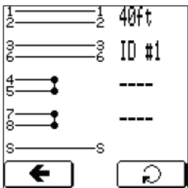
Разводка кабеля с перепуткой проводов между парами 4-5 и 7-8.
