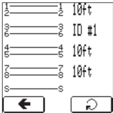
Хорошая разводка проводов
