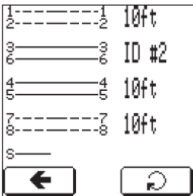
Разводка кабеля с разбивкой проводов между парами 1-2 и 7-8 и отсоединенным экраном.
