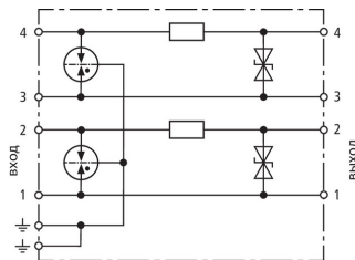
Принципиальная схема BVT MTTU 24
