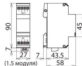
Размерный эскиз BVT MTTU 24
