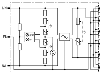
Принципиальная схема SFL PRO 6X 19"
