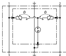
Принципиальная схема DR M 2P 30
