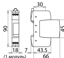
Размерный эскиз DR M 2P 30
