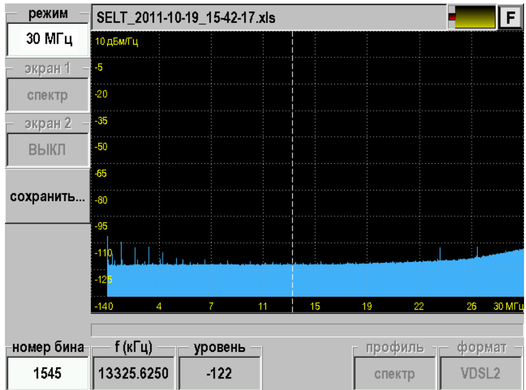
Рис. 26. 30 МГц.
