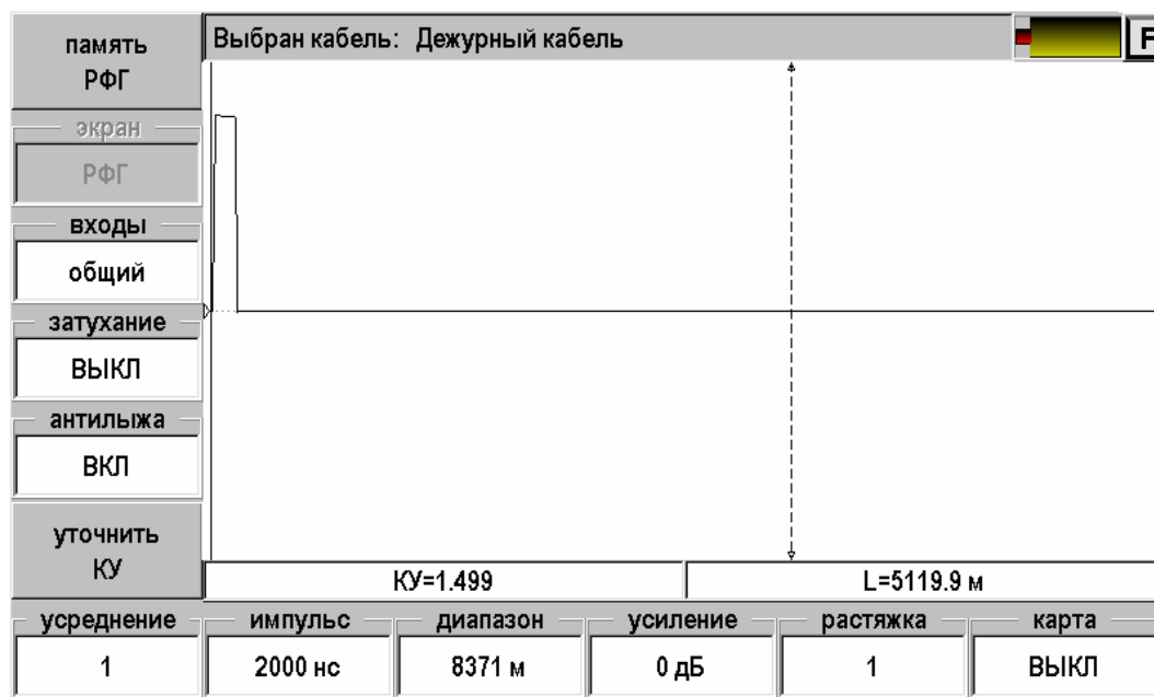
Рис. 31. Просмотр рефлектограммы.
