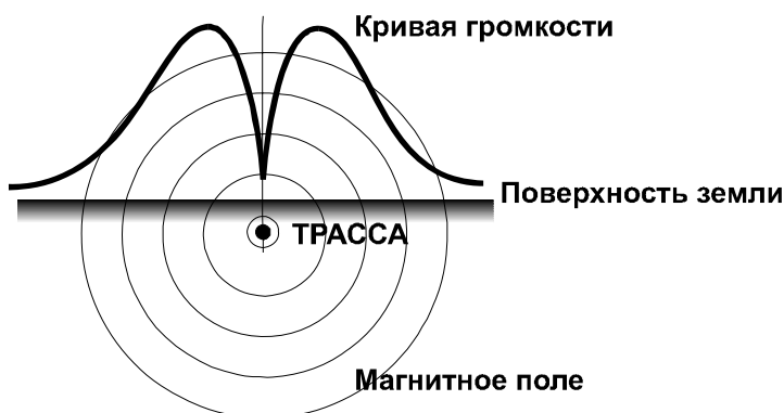
Рис.3 Поиск трассы по методу минимума.
