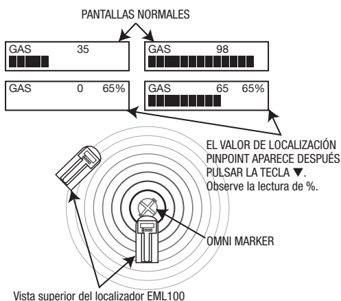
Figura 14. Característica Pinpoint
