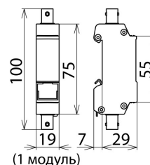
Размерный эскиз DGA BNC VCD
