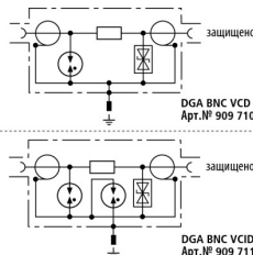
Принципиальная схема DGA BNC VCD
