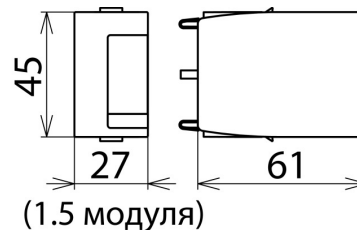
Размерный эскиз DG MOD E H LI 1000 (1.5 модуля)
