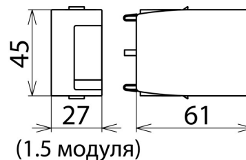
Размерный эскиз DG MOD E H LI 1000
