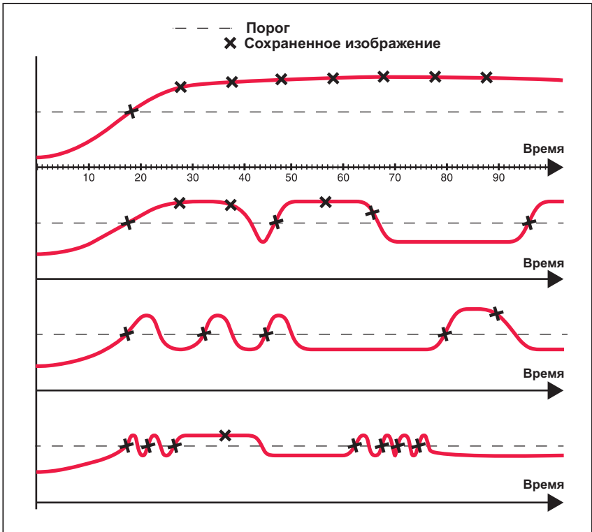
Рисунок 11. Сценарии захвата изображений для режима сигнализации автоматической проверки
