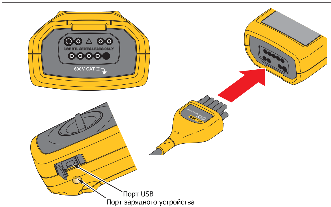
Рис. 1-2. Терминалы ввода-вывода
