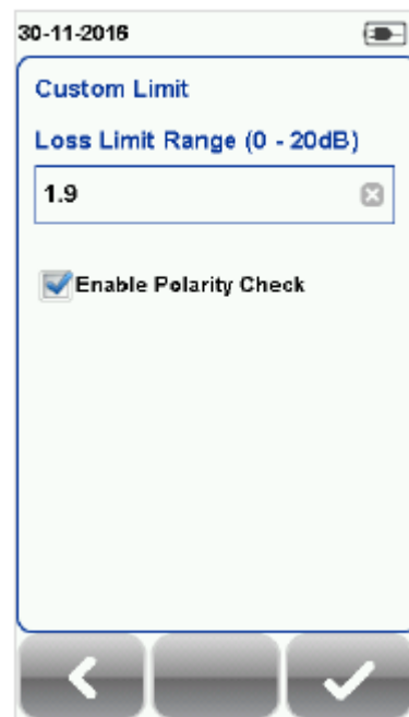
Использование пользовательских предельных условий с/без проверки полярности (Polarity Check).
