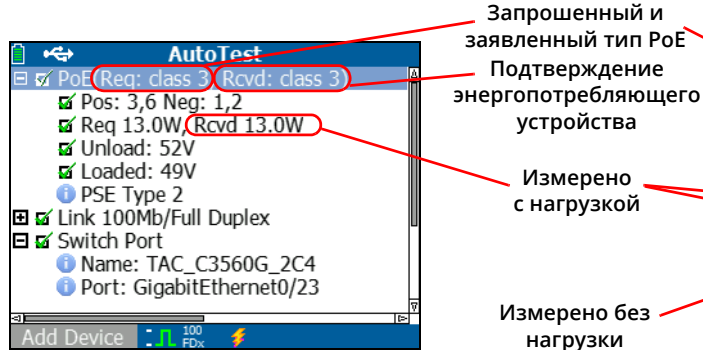
Рис.23. Результаты автотеста — функция PoE с использованием TruePower
