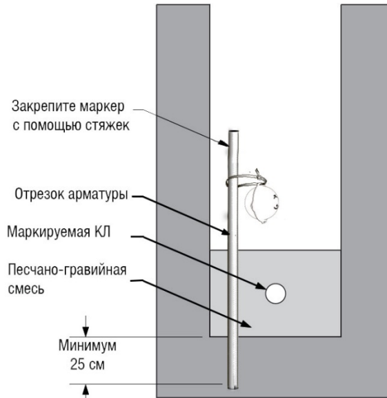
Рисунок 9 – Установка маркера OtiniMarker с креплением к вертикальному стержню
