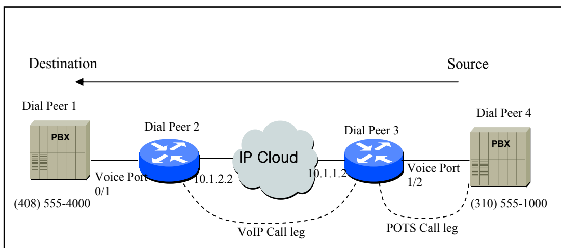
Figure 5.4 Исходящий звонок с точки зрения POTS Dial Peer 2
