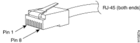
[Диаграмма D-1 Соединитель (коннектор) 10Base-T RJ-45 ]
