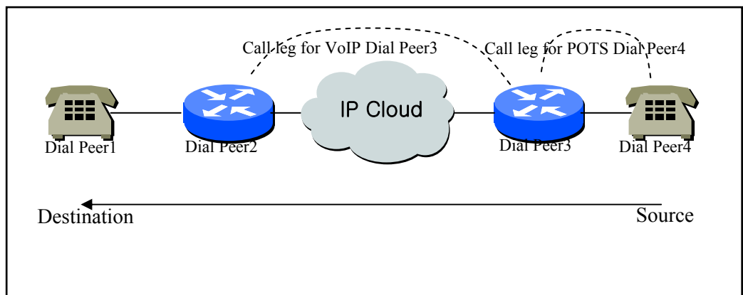
Figure 5-2: Участники звонка Dial Peer с точки зрения шлюза назначения
