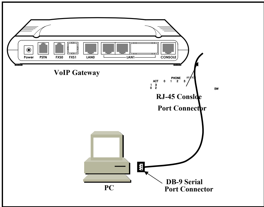
[Рис. 3.1 Подключение консольного кабеля]
