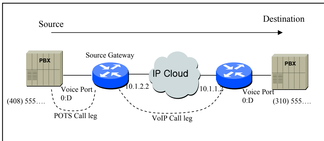
Figure 5.3 Исходящий звонок с точки зрения POTS Dial Peer 1
