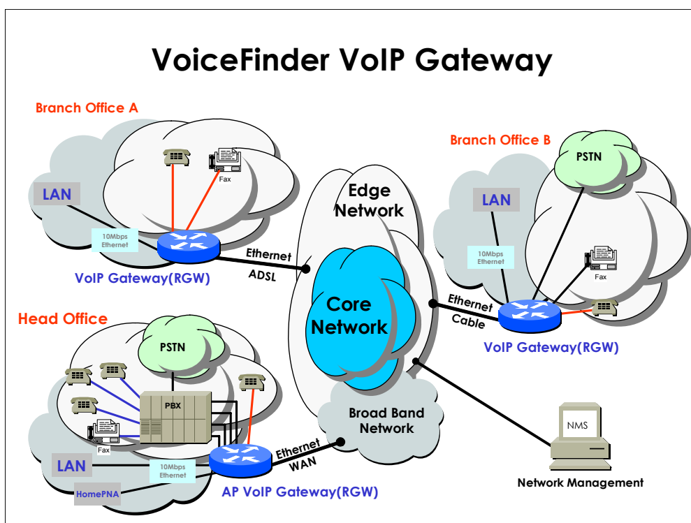
[ Рис. 1-1 Диаграмма межсетевого взаимодействия с использованием шлюза AddPac VoiceFinder ]
