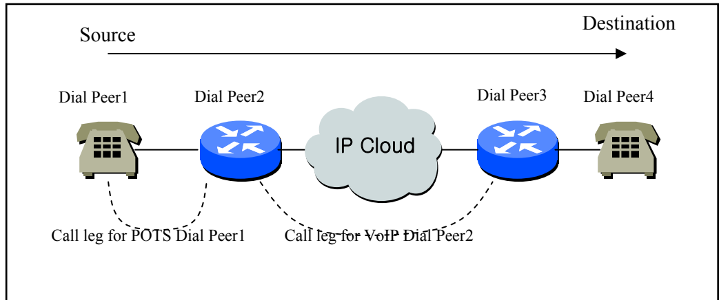
Figure 5-1: Участки звонка Dial Peer с точки зрения исходного шлюза
