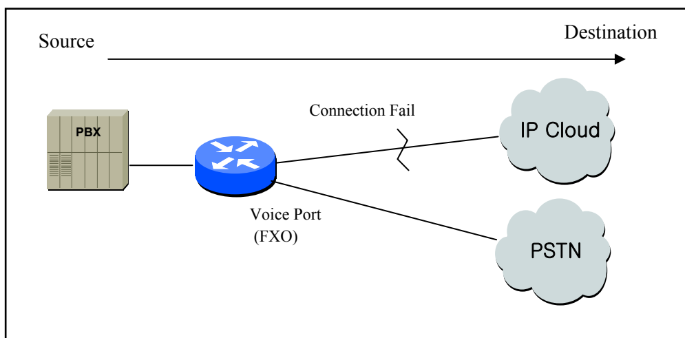
Figure 5.6 Изменение маршрута в ТфОП
